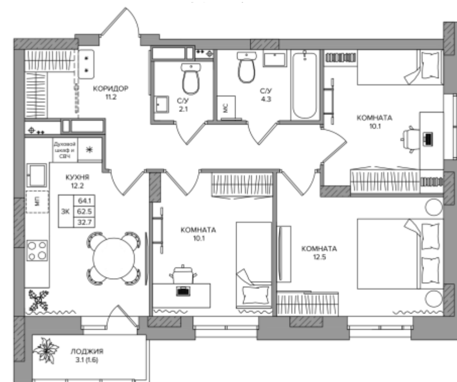
Секция 1 3-5, 7-16 этажи
